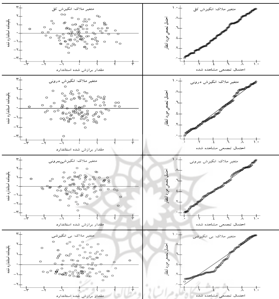
نمودار ۱. پراکنش مقادیر برازش شده استاندارد در مقابل باقیمانده‌های استاندارد شده (تعیین ثابت بودن واریانس) و پراکنش بین باقیمانده‌های مورد انتظار در مقابل باقیمانده‌ها (نمودار چندک-چندک نرمال) در مدل‌های رگرسیون خطی
