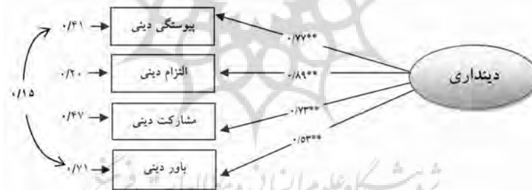
شکل ۱. مدل تحلیل عاملی دین‌داری
