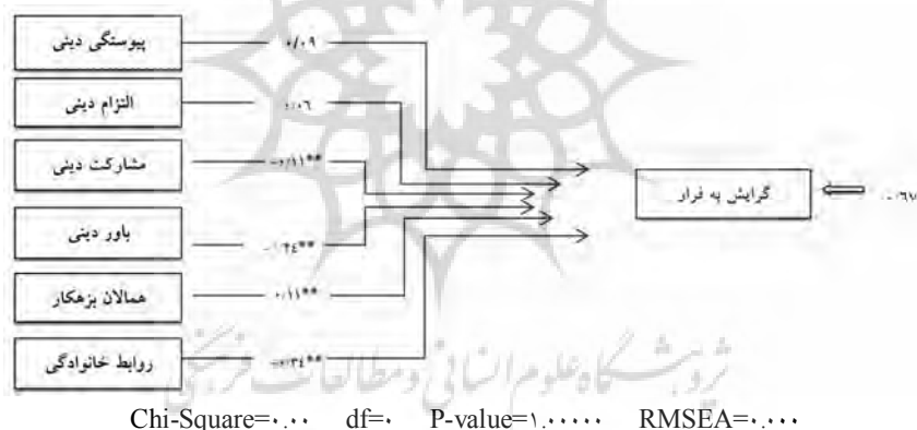
شکل ۵. مدل تحلیل رگرسیونی
