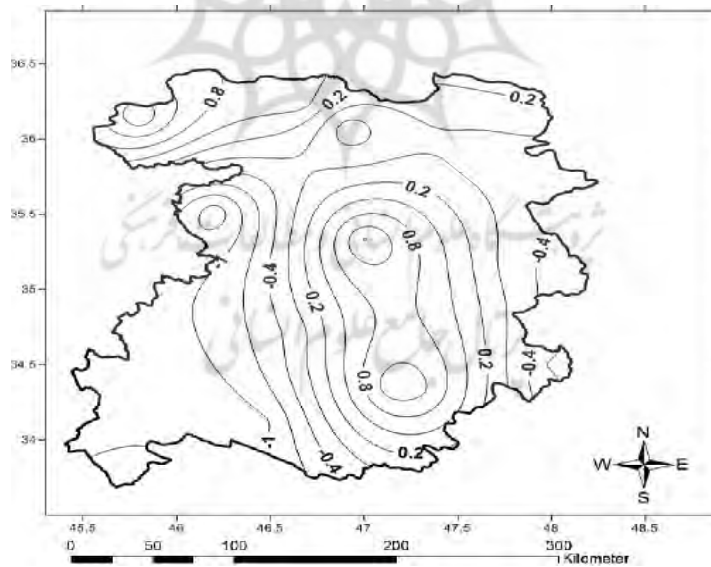
شکل (۵) قلمرو مکانی نمرات عامل ابرناکی
