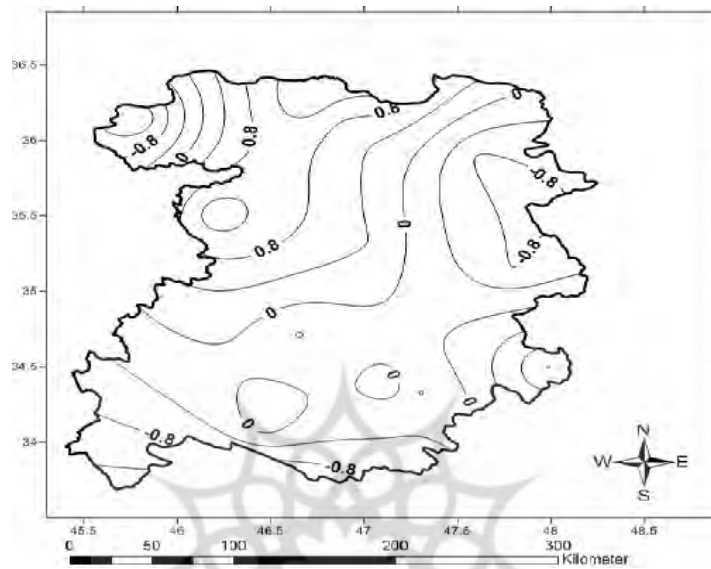
شکل (۴) قلمرو مکانی نمرات عامل رطوبت
