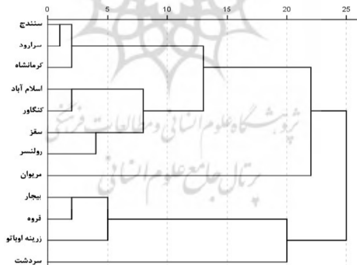
شکل (۹) دارنمای اقلیمی ایستگاه‌های منطقه مورد مطالعه
