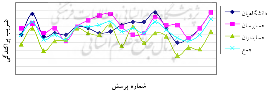
شکل (۳): ضریب پراکندگی پرسش‌های بعد اقتصادی از نظر گروه‌های پرسش
