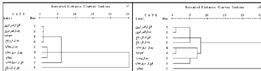
شکل (۵) نمودار درختی تجزیه و تحلیل خوشه‌ای شاخص‌های کیفیت آب (الف) و فلزات سنگین (ب) ایستگاه‌های مختلف رود الوند
