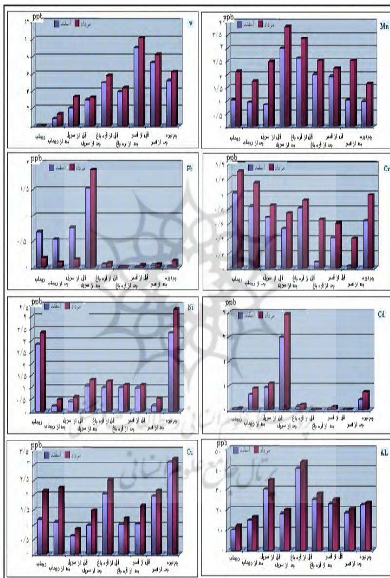
شکل (۳) تغییرات مکانی فلزات سنگین در امتداد رود الوند در دو ماه مرداد و اسفند
