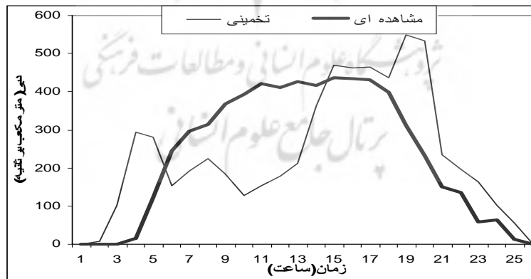
شکل (۱۰) هیدروگراف واحد مشاهداتی و تخمینی (۷۳/۱۰/۲۸)
