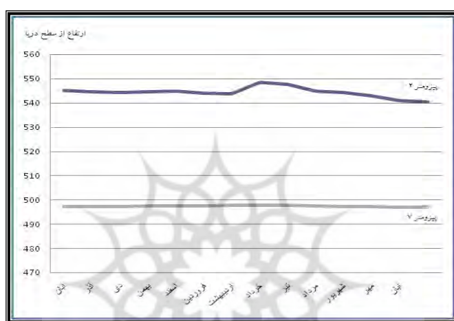
شکل ۶- مقایسه گراف‌های ماهانه پیزومترهای شماره ۲ و ۷
