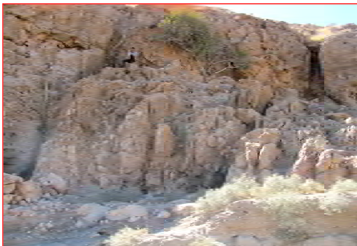
شکل ۴: درز و شکستگی‌های موجود در منطقه (غرب روستای دارج بالا)
