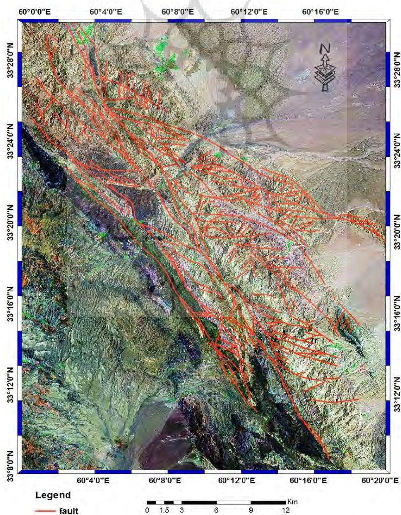
شکل ۵: نقشه پراکندگی گسل‌ها و شکستگی‌های موجود در سنگ‌های کربناته منطقه مورد مطالعه
