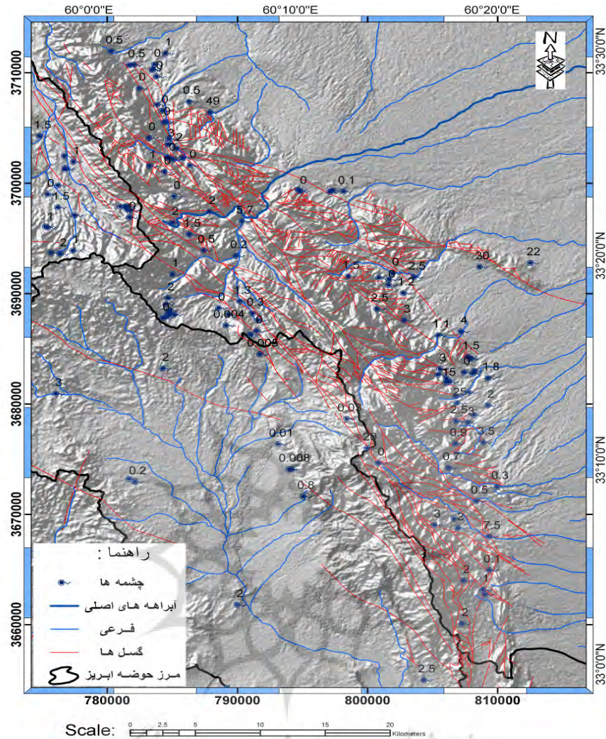
شکل ۱۰: نقشه موقعیت چشمه‌های موجود در منطقه
