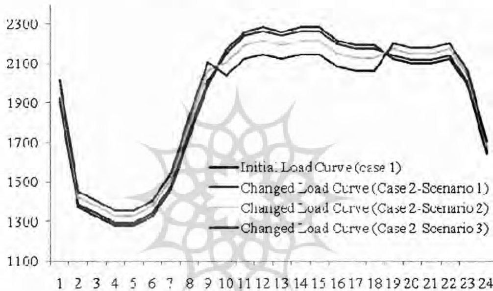
شکل (۴) منحنی بار اولیه و تغییر یافته برای شبکه ۲۴ شین IEEE-RTS با پتانسیل‌های مختلف اجرای پاسخ‌گویی بار اضطراری (EDRP)
