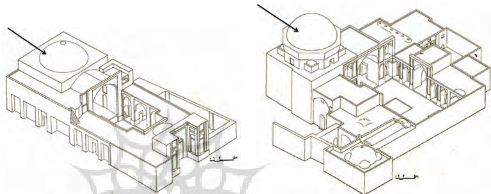
تصویر ۱۳: گنبدخانه در مدرسه شیخ ابوالقاسم طراز در یزد (حاجی قاسمی ۱۳۷۹)
