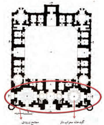
تصویر ۱۵: تهرانگ مدرسه غیاثیه (حاجی قاسمی ۱۳۷۹، ۱۱۴)
