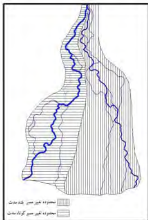
شکل ۱۷: پهنه‌های در معرض حرکات پیچان رودی و تغییر مسیر در سطح دلتای حسن لنگی شکل ۱۸: پهنه‌های در معرض حرکات پیچان رودی و تغییر مسیر در سطح دلتای شور
