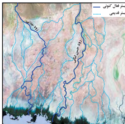
شکل ۵: مسیر فعال و بسترهای قدیمی در سطح دلتای مرکب رودخانه‌های حسن لنگی و جلابی. تغییر مسیرهای جدیدتر در سطح این دلتا نسبت به سایر دلتاها کمتر است.
