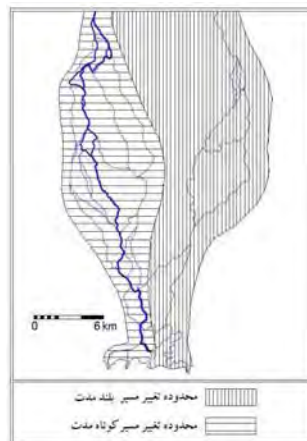
شکل ۱۷: پهنه‌های در معرض حرکات پیچان رودی و تغییر مسیر در سطح دلتای حسن لنگی شکل ۱۸: پهنه‌های در معرض حرکات پیچان رودی و تغییر مسیر در سطح دلتای شور
