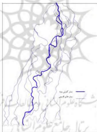
شکل ۱۹: پهنه‌های در معرض حرکات پیچان رودی و تغییر مسیر در سطح دلتای جلابی
