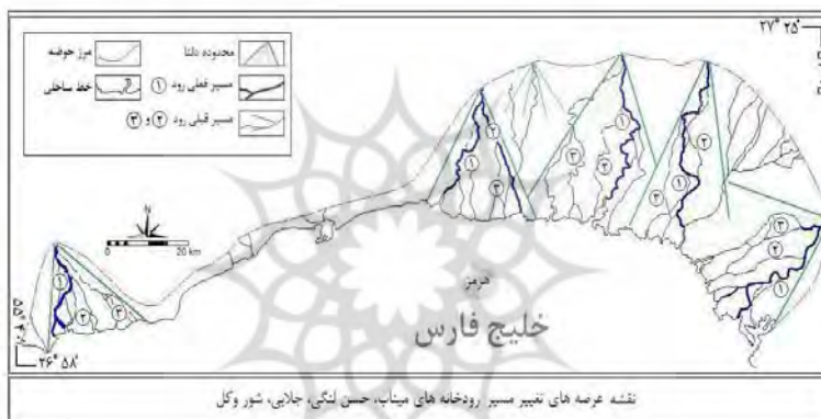
شکل ۲۰: محدوده تغییر مسیر رودخانه‌های شور، جلابی و حسن لنگی
