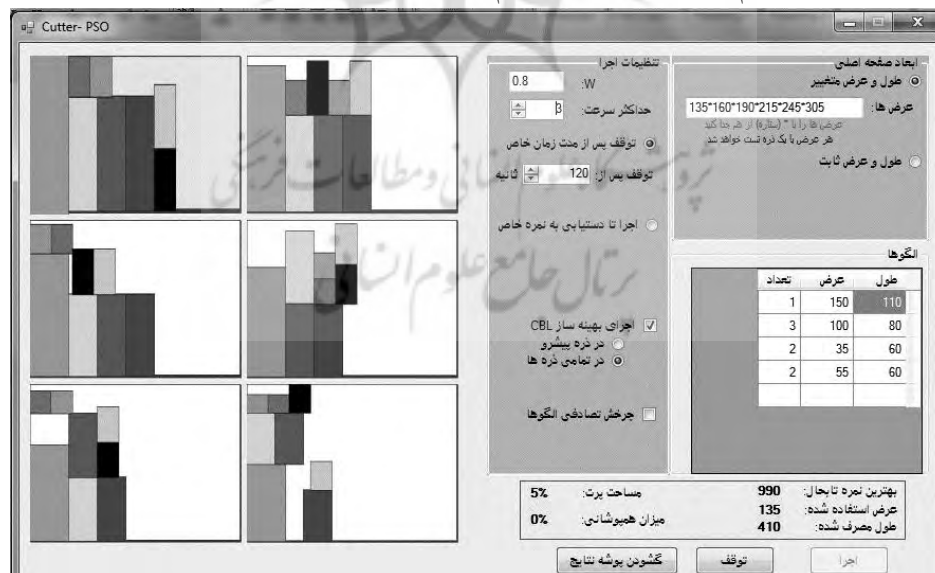
شکل ۷. اعمال الگوریتم CUL روی تمام ذره‌ها
