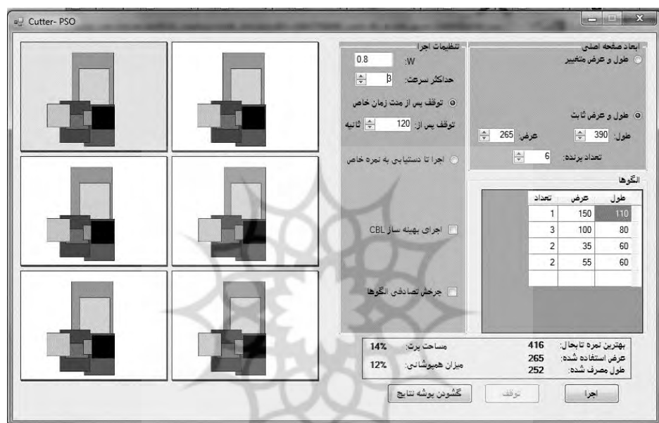
شکل ۵. اجرای الگوریتم پیشنهادی در صورت عدم اعمال الگوریتم CUL
