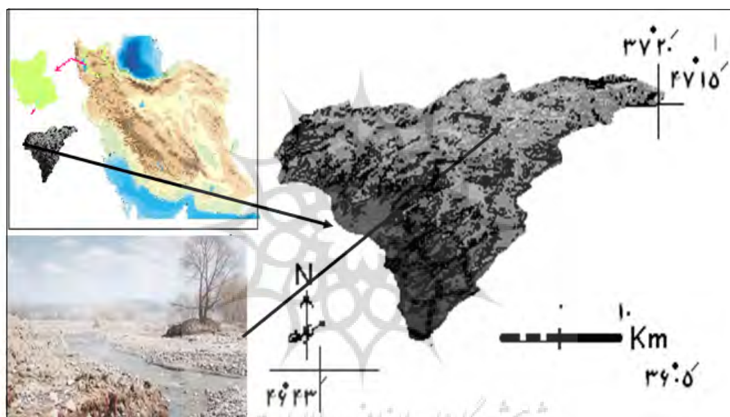
شکل ۱: موقعیت جغرافیایی حوضه‌ی رودخانه شور و تصویری از پیچان در مسیر جریان آن
