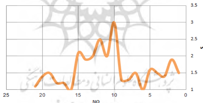
شکل ۴: میزان سینوزیته رودخانه‌ی شورچای از محل سد ملاجیغ (قطعه شماره ۲۱) تا محل اتصال آن به رودخانه قرنقو (قطعه شماره ۱).
