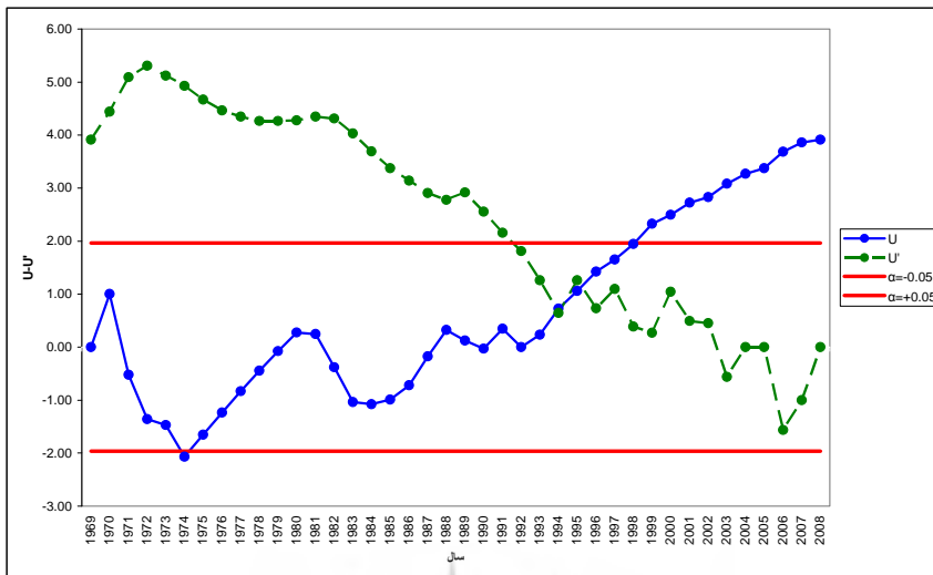
شکل شماره ۲- نمودار تغییرات U و U' میانگین دمای حداقل ایستگاه سینوپتیک سنندج
