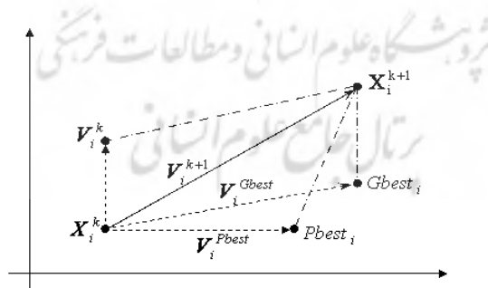
شکل ۱. نحوه تحول سرعت و مکان ذرات در PSO
