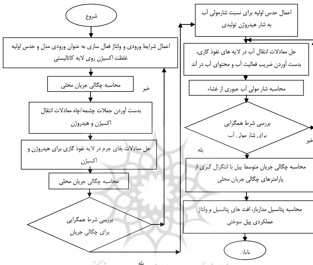
شکل ۵: الگوریتم حل
