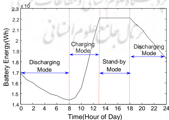
شکل ۱۰: تغییرات انرژی باتری در یک شبانه روز
