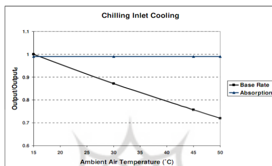
شکل ۱۴: تاثیر سیستم تبرید جذبی با دمای خروجی C ۱۵ بر عملکرد توربین گازی
