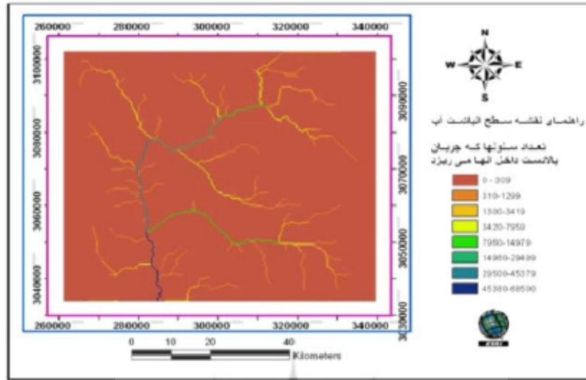
شکل ۶: نقشه سطح انباشت آب حوضه دامن مأخذ: نگارندگان
