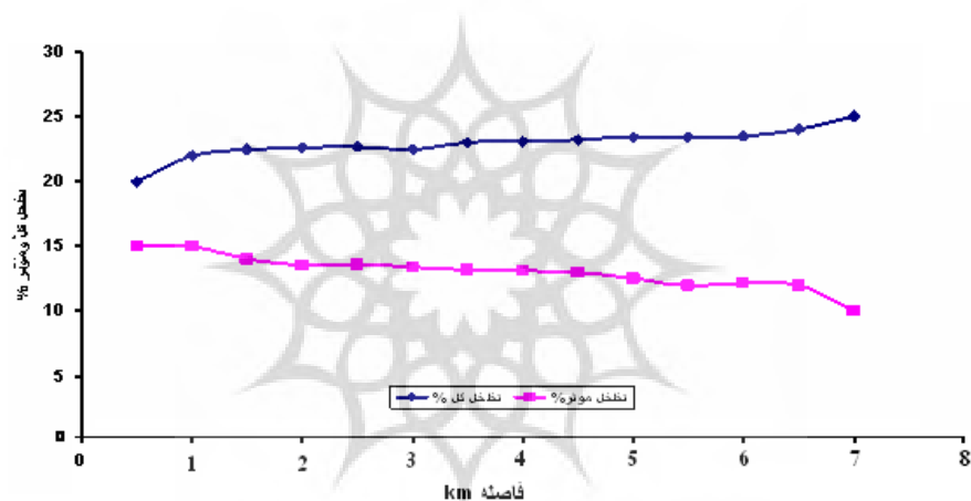
شکل ۶- دیاگرام تغییرات تخلخل کل و موثر رسوبات آبرفت رودخانه در آبراهه اصلی
