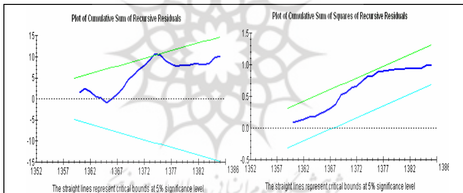
نمودار ۳. آزمون‌های پایداری مدل ARDL(1, 1, 0, 0) بدون لحاظ شکست و متغیر وابسته IGDP
