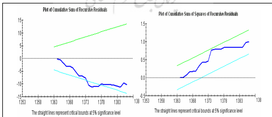
نمودار ۴. آزمون‌های پایداری مدل ARDL(1, 2, 2, 0) بدون لحاظ شکست و متغیر وابسته IELC
