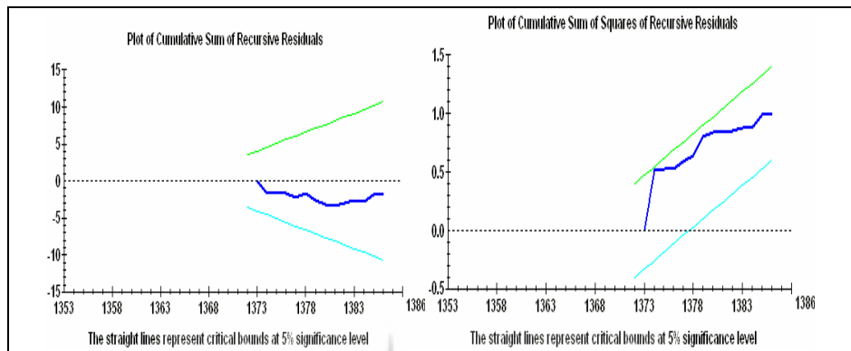
نمودار ۲. آزمون‌های پایداری مدل ARDL(1, 2, 2, 0) با لحاظ شکست و متغیر وابسته IELC
