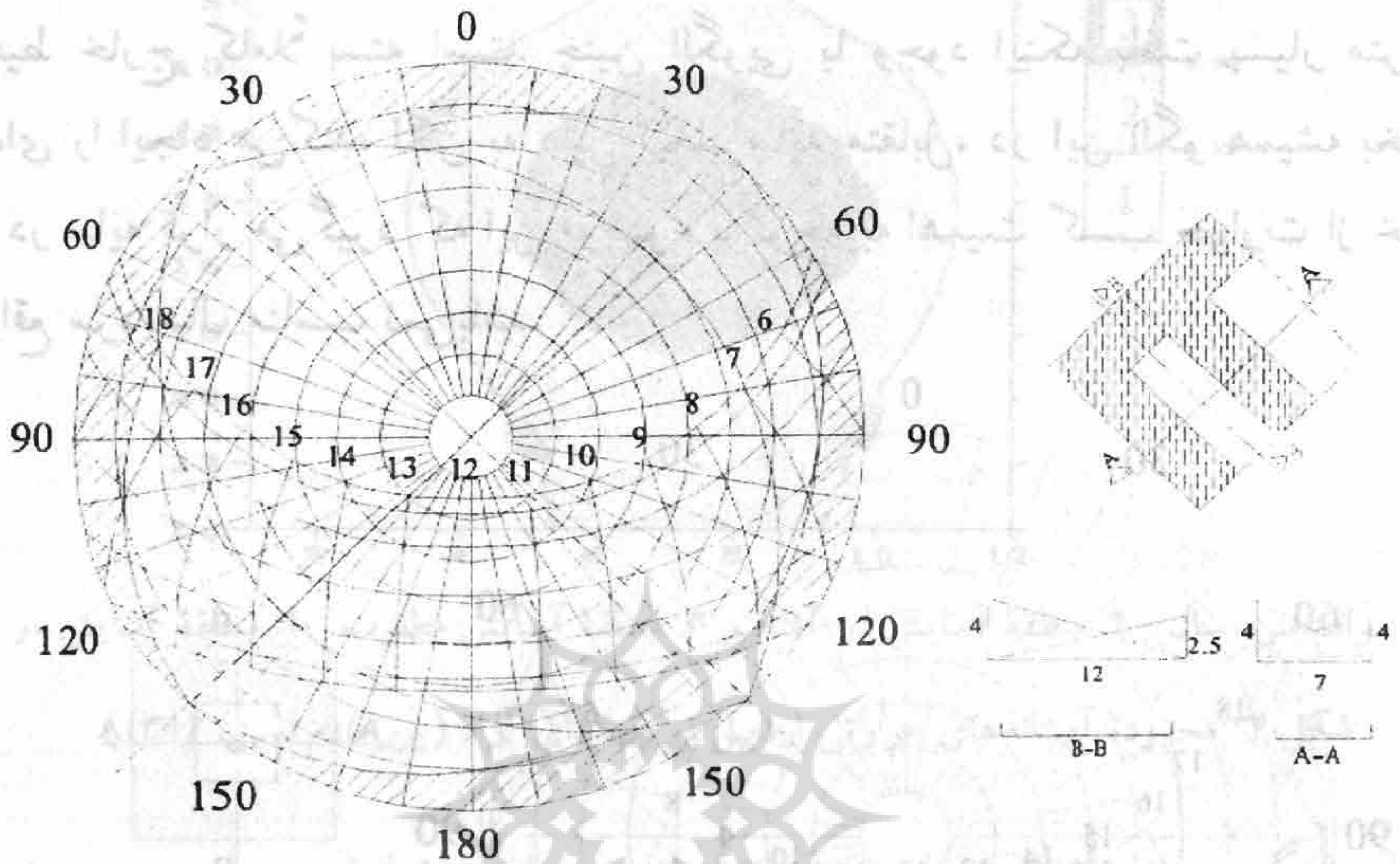
شکل ۴ موقعیت حیاط مورد نظر بر روی دیاگرام مسیر حرکت خورشید (پورخادم نمین، ۱۳۸۲)
