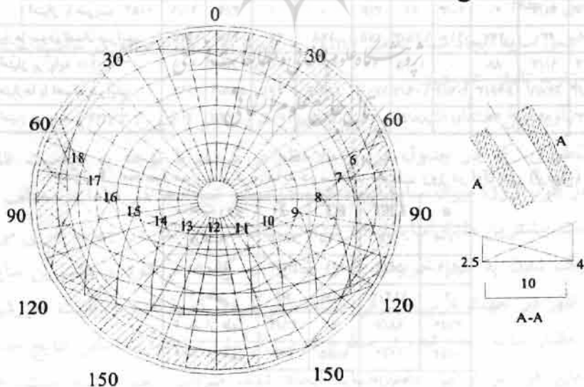
شکل ۸ موقعیت مسیر ارتباطی مورد نظر بر روی دیاگرام مسیر حرکت خورشید (پورخادم نمین، ۱۳۸۲)
