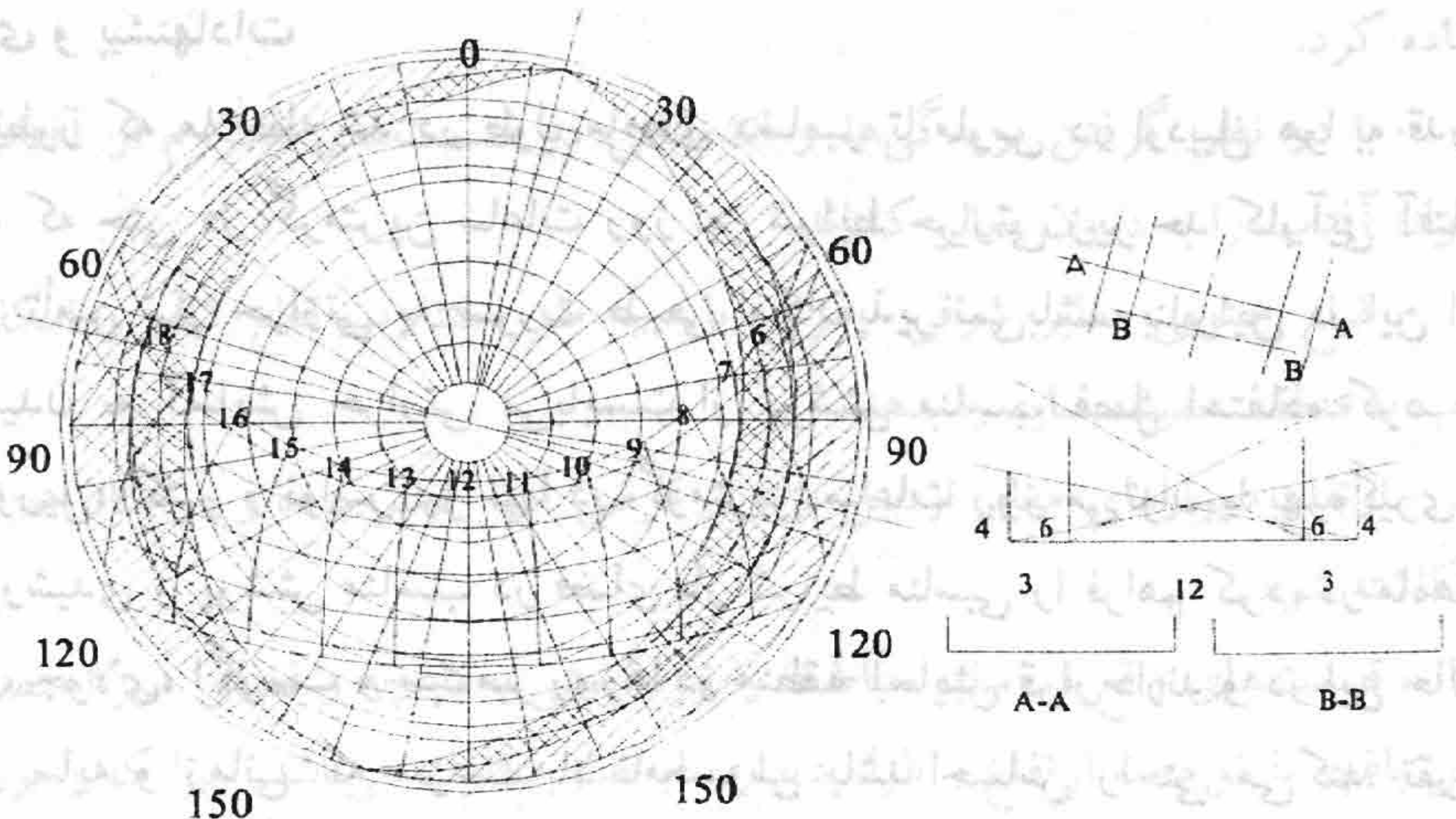
شکل ۱۰ موقعیت مسیر ارتباطی مورد نظر بر روی دیاگرام مسیر حرکت خورشید (پورخادم نمین، ۱۳۸۲)
