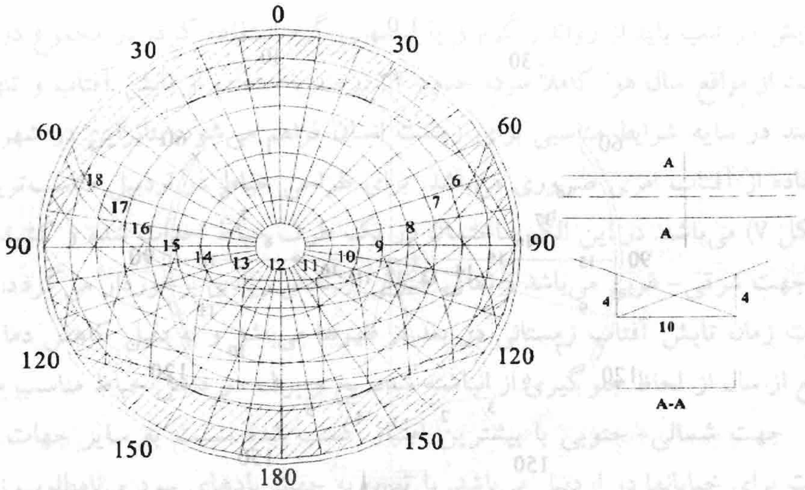
شکل ۹ موقعیت مسیر ارتباطی مورد نظر بر روی دیاگرام مسیر حرکت خورشید (پورخادم نمین، ۱۳۸۳)
