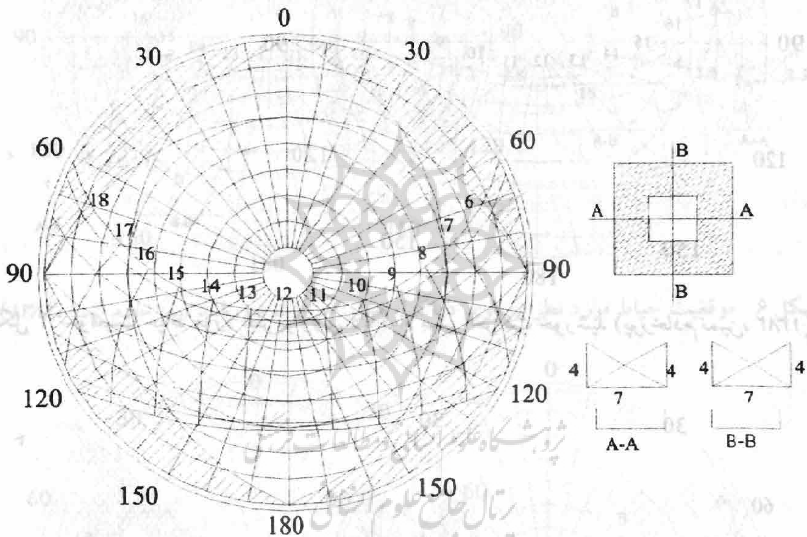
شکل ۳ موقعیت حیاط مورد نظر بر روی دیاگرام مسیر حرکت خورشید (پورخادم نمین، ۱۳۸۲)
