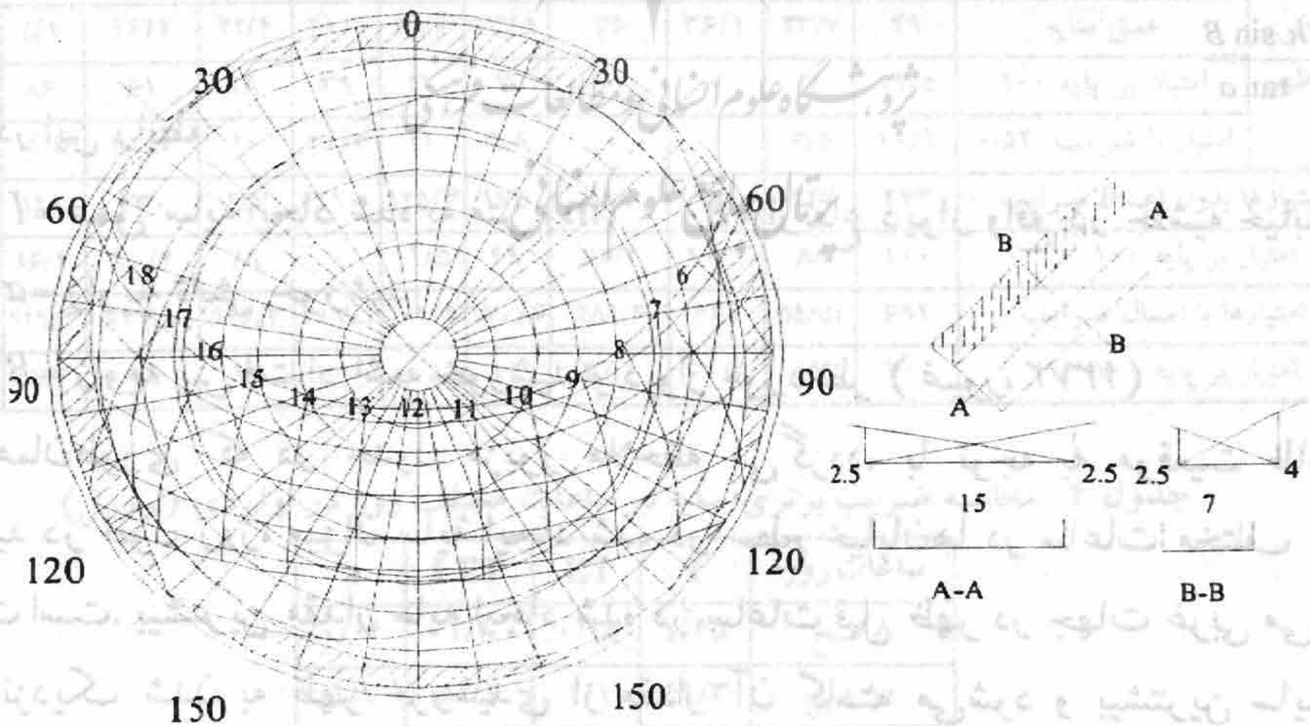
شکل ۷ موقعیت حیاط مورد نظر بر روی دیاگرام مسیر حرکت خورشید (پورخادم نمین، ۱۳۸۲)
