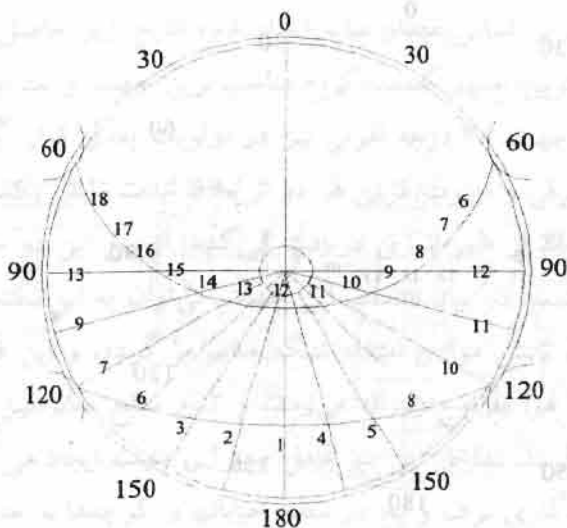
شکل ۱۱ ترتیب اولویت جهت معابر از نظر کاهش میزان سایه در سطح خیابانها در فصل زمستان (پورخادم تمین، ۱۳۸۴)
