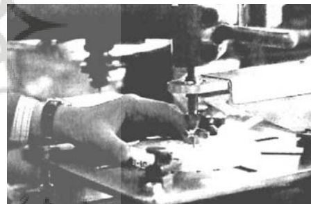
تصویر ۲۷- حکاکی توسط پانتوگراف از روی نمونه گچی
