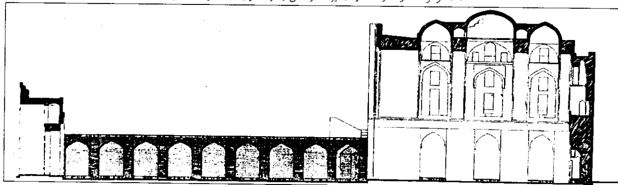
لوحة شماره ۱۱- برش طولی مسجد جامع قاین - دیده به شرق ماخذ مرکز اسناد و مدارک سازمان میراث فرهنگی و گردشگری استان خراسان رضوی
