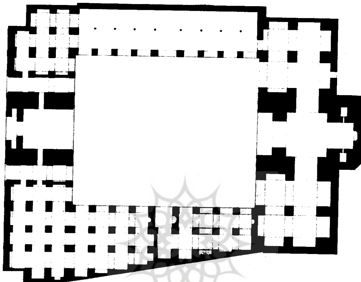
لوحة شماره ۱- پلان مسجد جامع شرقی مآخذ مرکز اسناد و مدارک سازمان میراث فرهنگی و گردشگری استان خراسان رضوی
