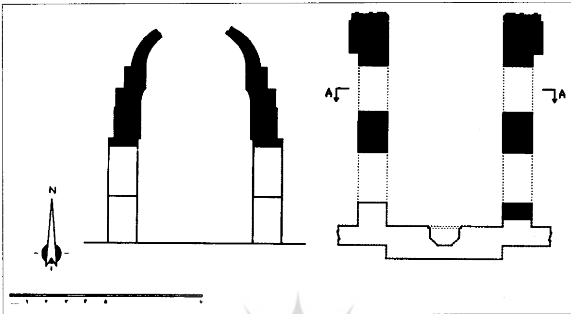
لوحة شماره ۶- پلان و برش مسجد خسرو و شیر ماخذ مرکز اسناد و مدارک سازمان میراث فرهنگی و گردشگری استان خراسان رضوی
