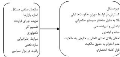
شکل شماره (3) - نگاشت مشخصه‌های اجزای بردار حالت حقوق مالکیت جامعه ایران در قرن بیستم
