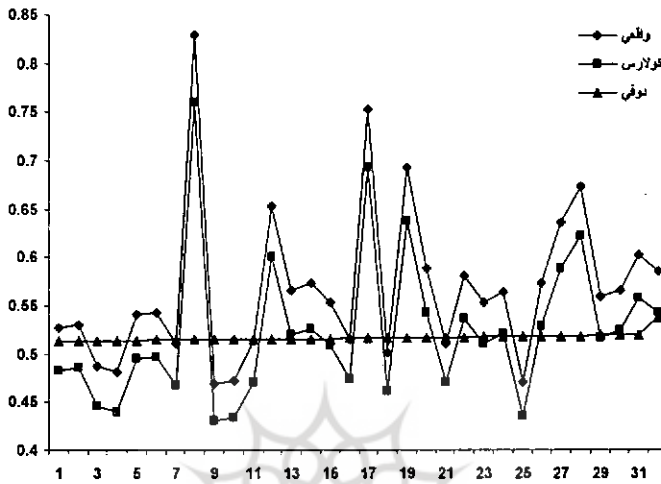
شکل (۳) نمودار ضریب صافی هوا برای ماه ژانویه به صورت روزانه (بندرعباس)
