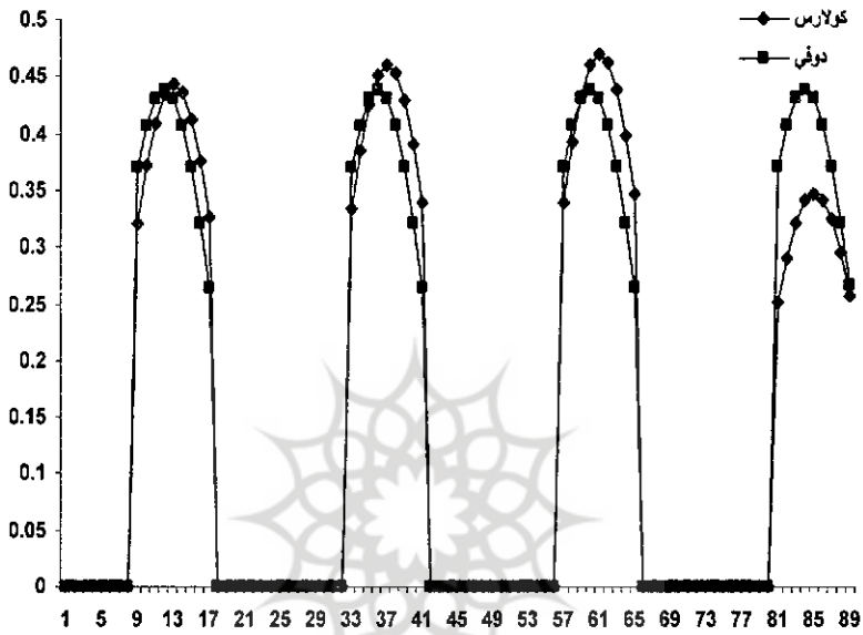
شکل (۵) نمودار ضریب صافی هوا برای ۴ روز اول ماه ژانویه به صورت ساعتی (تبریز)
