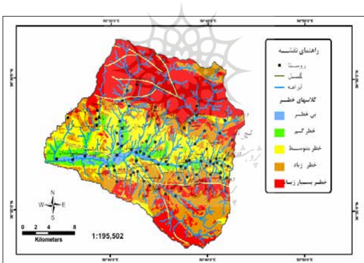
شکل ۱۲. نقشه پهنه‌بندی خطر زمین لغزش با مدل ارزش ا اطلاعاتی آبخیز باغدشت
