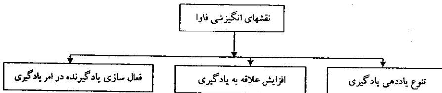
نمودار ۳- نقش‌های انگیزشی فاوا در فرایند یاددهی یادگیری
