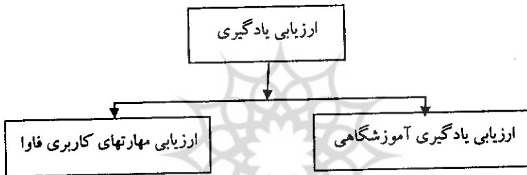
نمودار ۵- نقش فاوا در ارزیابی یادگیری
