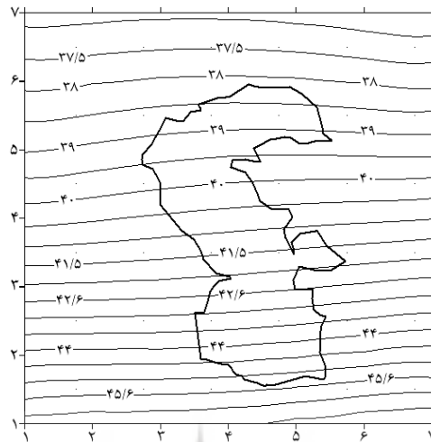
شکل ۶ نقشه مقادیر همدمای پتانسیل کل لایه جوی ۱۰۰۰ تا ۱۰۰ هکتوپاسکال برحسب درجه سانتی گراد در محدوده خزر
