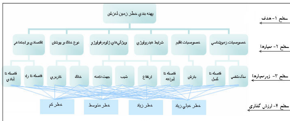
شکل (۲) ساختار سلسله مراتب AHP برای پهنه‌بندی خطر زمین لغزش
