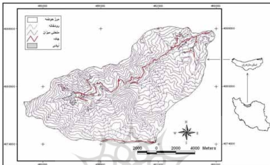
شکل (۱) نقشهٔ مورفومتریک جغرافیایی حوضه‌ی صفارود
