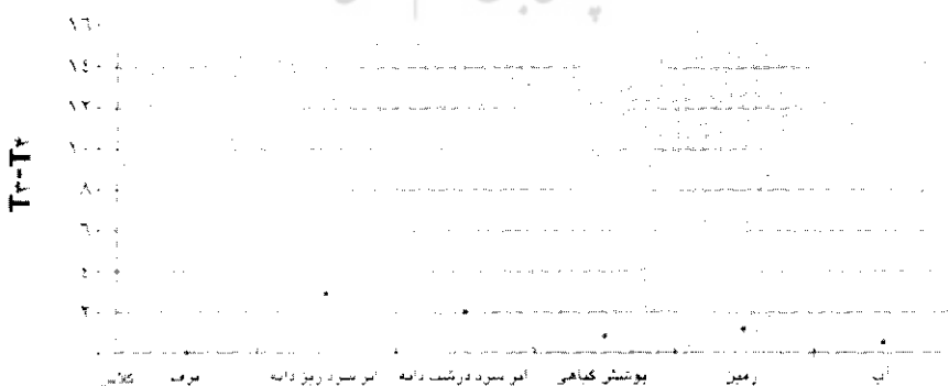
نمودار ۱ مقایسه پدیده‌های مختلف از نظر مقدار شاخص T_r - T_p (تصویر ۲۵/۱/۲۰۰۰)
