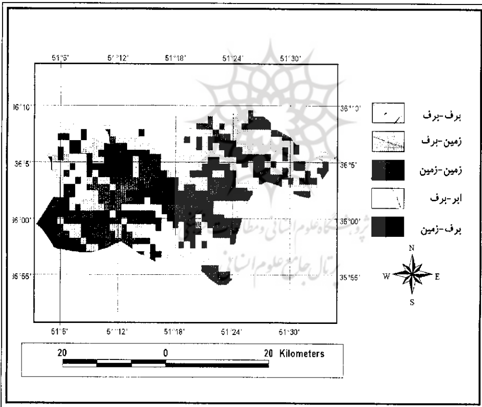
تصویر ۵ نقشه تغییرات پوشش برف که از تفریق تصاویر مربوط به (۲۰۰۰/۰۱/۲۵) و (۲۰۰۰/۰۲/۱۲) تهیه شده است.
