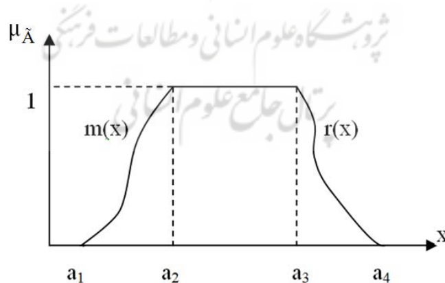
نمودار ۱. اعداد فازی
