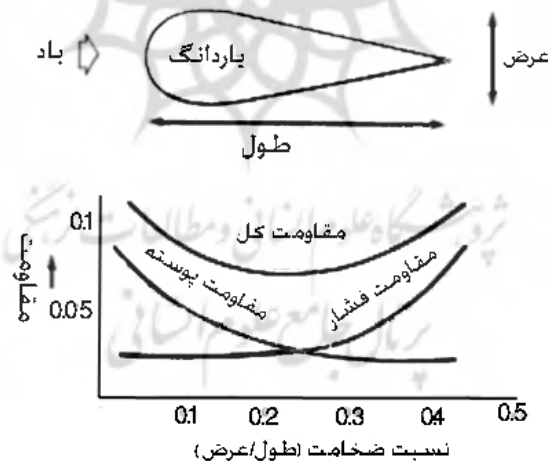
شکل ۱. نمودار وضعیت آئروپدینامیکی یاردانگ‌ها. زمانی مقاومت کل در برابر باد حداقل است که نسبت عرض به طول در حدود ۲۵/۱ باشد.
