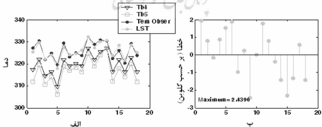
شکل ۳. نتایج حاصل از اعمال مدل LST بر روی داده‌های ماهواره‌ای و مقایسه نتایج آن با داده‌های هواشناسی (الف)، میزان خطای مدل LST در مقایسه با داده‌های هواشناسی (ب)
