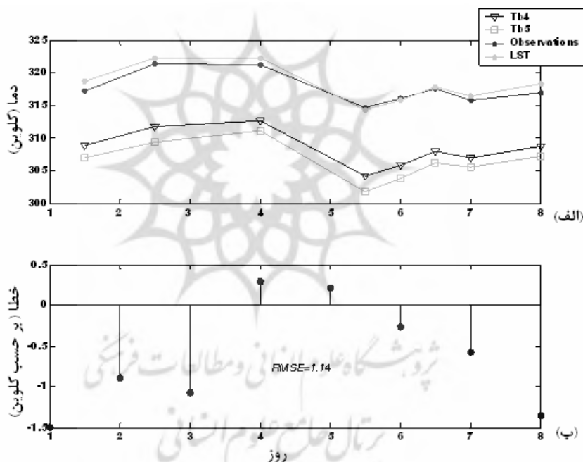
شکل ۴. (الف) مشاهدات زمینی، T_{b4} و T_{b5} مربوط به آنها و نتایج حاصل از اعمال مدل LST بر روی آنها، (ب) میزان خطا برحسب کلون
