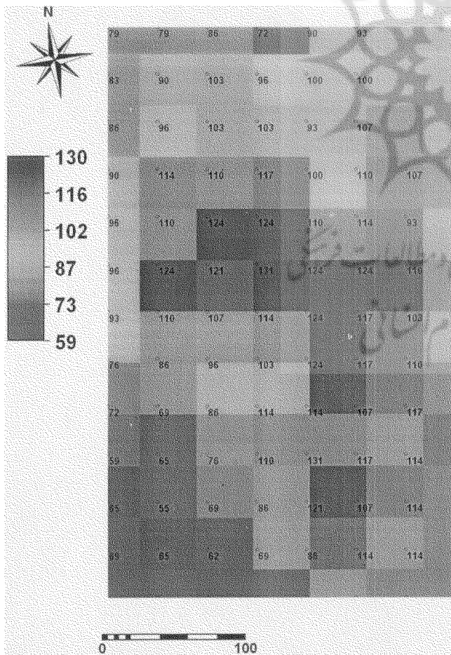
نگاره ۳: نقشه میزان رشد ذرت در قطعات مختلف مزرعه براساس شاخص NDVI
