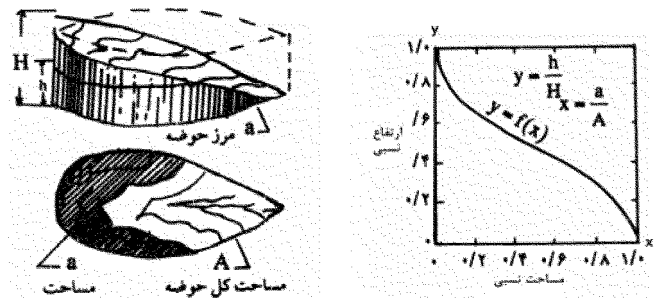
نگاره ۲: منحنی هیپسومتری بی بعد
