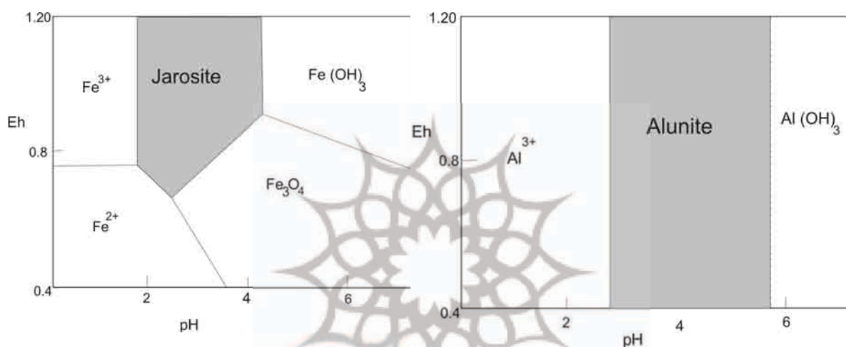
شکل ۸. شرایط پایداری ژاروسیت که تابع دو عامل Eh و pH است [۱۶].
