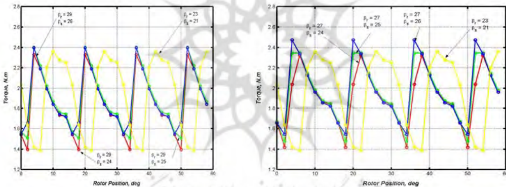
شکل ۵: مقایسه گشتاور چهار فاز با تغییرات زوایای قطب رتور و استاتور شکل ۶: مقایسه گشتاور چهار فاز با تغییرات زوایای قطب رتور و استاتور
