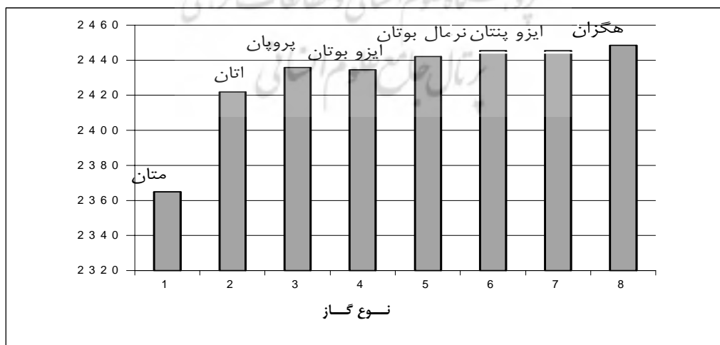
شکل ۱: مقایسه دمای شعله آدیباتیک گازهای تشکیل دهنده گاز طبیعی
