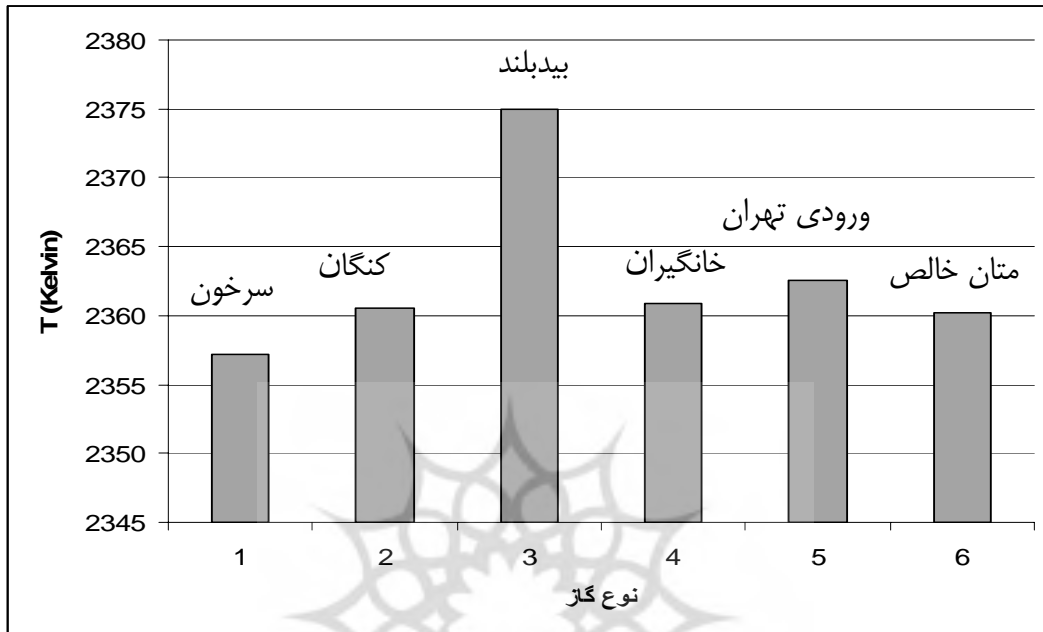
شکل ۲: مقایسه دمای شعله آدیاباتیک حوزه های گاز ایران (دما ۵۰ درجه و استوکیومتریک)
