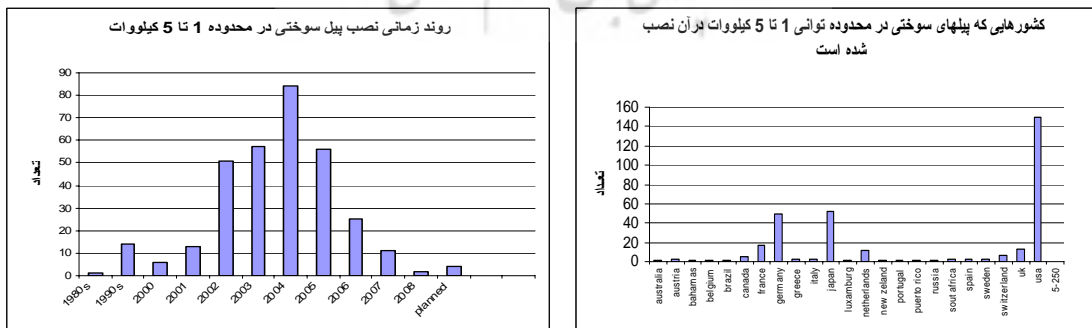
شکل (۱۵و۱۴): روند زمانی و محل نصب پیل‌های سوختی نصب شده در محدوده توانی ۱ تا ۵ کیلووات
