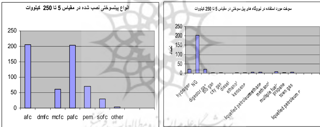
شکل (۱۳و۱۲): سوخت‌های مورد استفاده و انواع پیل‌های سوختی نصب شده در محدوده توانی ۵ تا ۲۵۰ کیلووات
