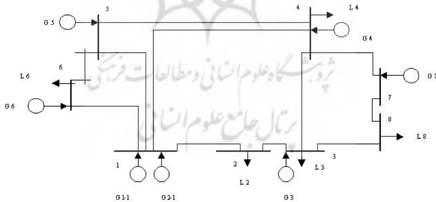
شکل ۲- شبکه نمونه
