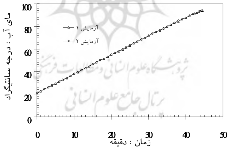
نمودار ۲- زمان جوش آمدن آب به میزان ۱۸۰۰۰ واتیمتر مکعب در سماور برقی ۳۰ لیتری تجاری
