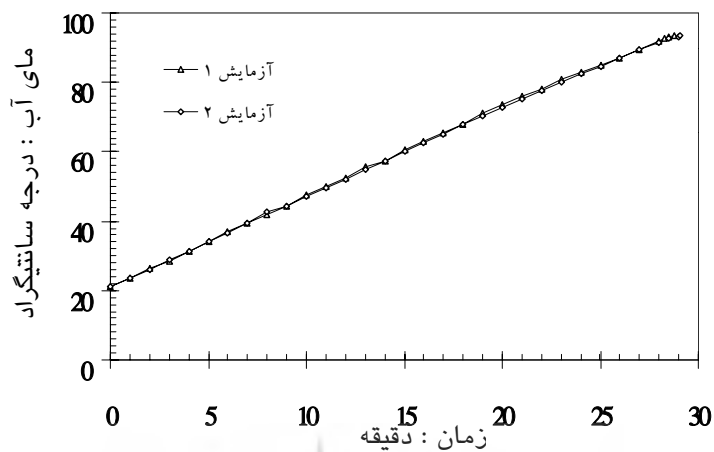
نمودار ۱- زمان جوش آمدن آب به میزان ۵۴۰۰ واتیمتر مکعب در سماور برقی ۶ لیتری خانگی
