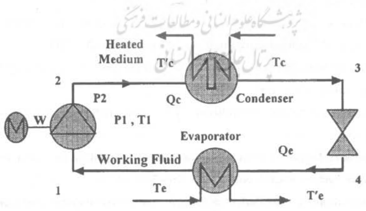
شکل ۲: نمایش یک سیکل پمپ حرارتی روی نمودار فشار - انتالپی
