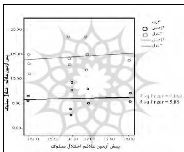
نمودار (۱) پراکندگی رابطه‌ی بین پیش‌آزمون و پس‌آزمون علایم اختلال سلوک
