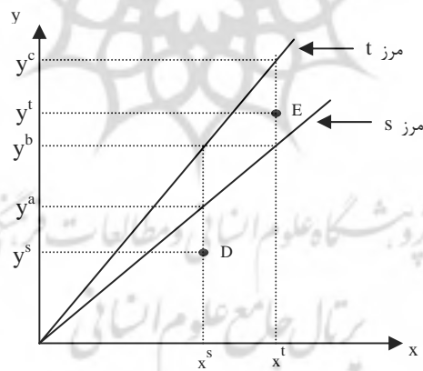
شکل ۴. تجزیه بهره‌وری شاخص مالکونیست (FGLR)
