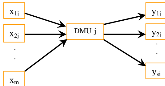
شکل ۱. نماد تصویری DMUj
