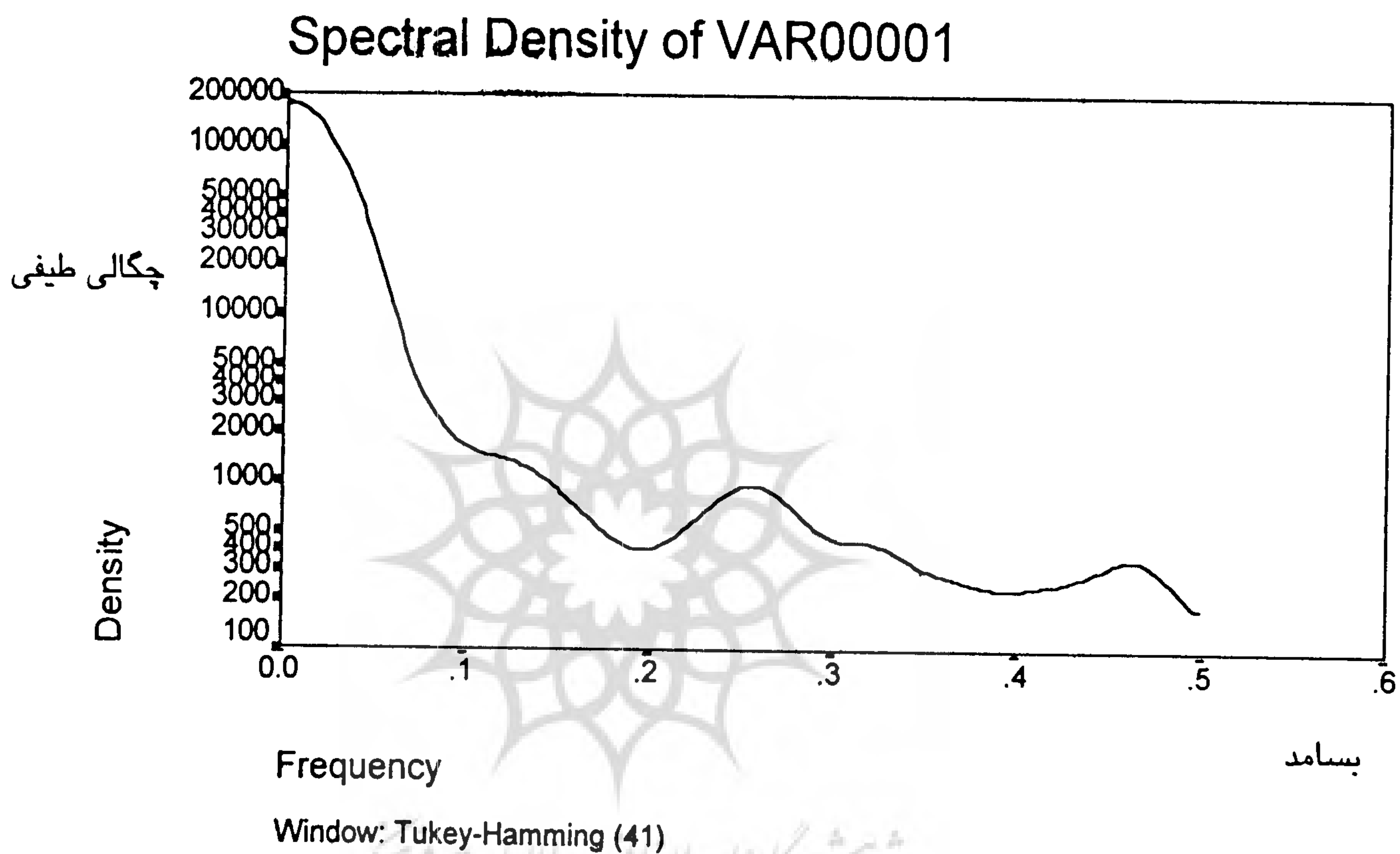
شکل شماره ۴ - تابع چگالی طیف داده‌های خام با پنجره توکی
