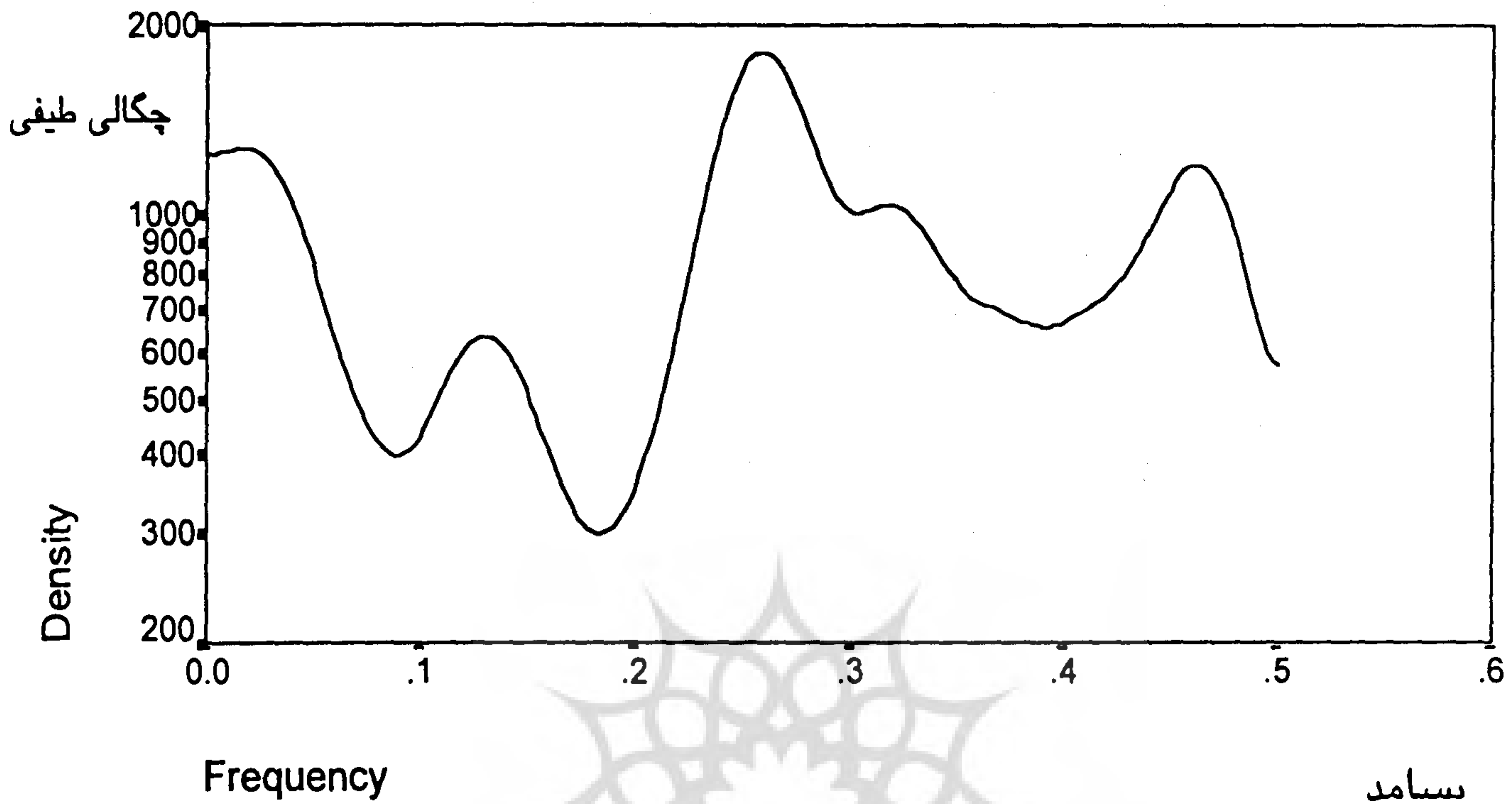
شکل شماره ۱۰ - تابع چگالی طیفی برای M=41
