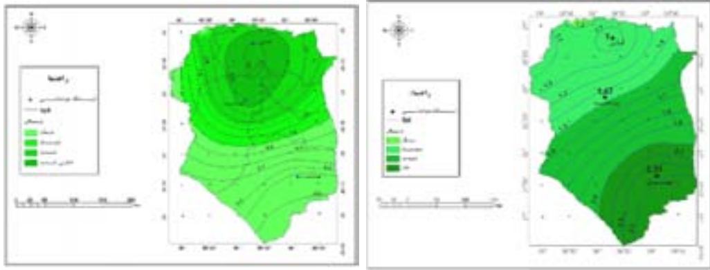
شکل ۱۸: تغییرات شدت ترسالی در استان خراسان جنوبی در سال ۱۹۸۶
