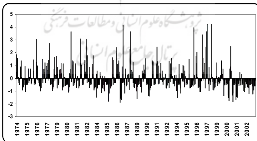
شکل ۶: نمودار تغییرات شاخص SPI فصلی استان خراسان جنوبی دوره‌ی آماری ۱۹۷۴-۲۰۰۳
