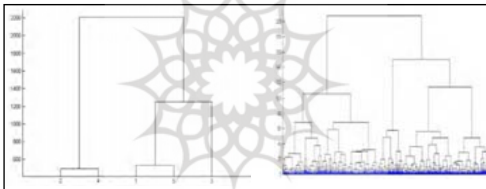
شکل ۱: نمودار درختی حاصل از تحلیل خوشه‌ای تیپ‌های همدید اصلی ایستگاه سنندج هوا با یکدیگر
