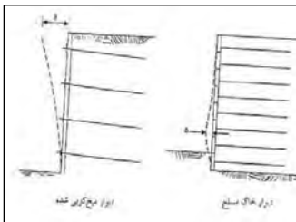
تصویر ۱۴- رفتار سیستم میخ کوبی. تصویر ۱۵- تفاوت تغییر مکان در دیوارهای خاک مسلح و دیوارهای میخ کوبی. مأخذ: (CLOUTERRE, 1991, 26)
