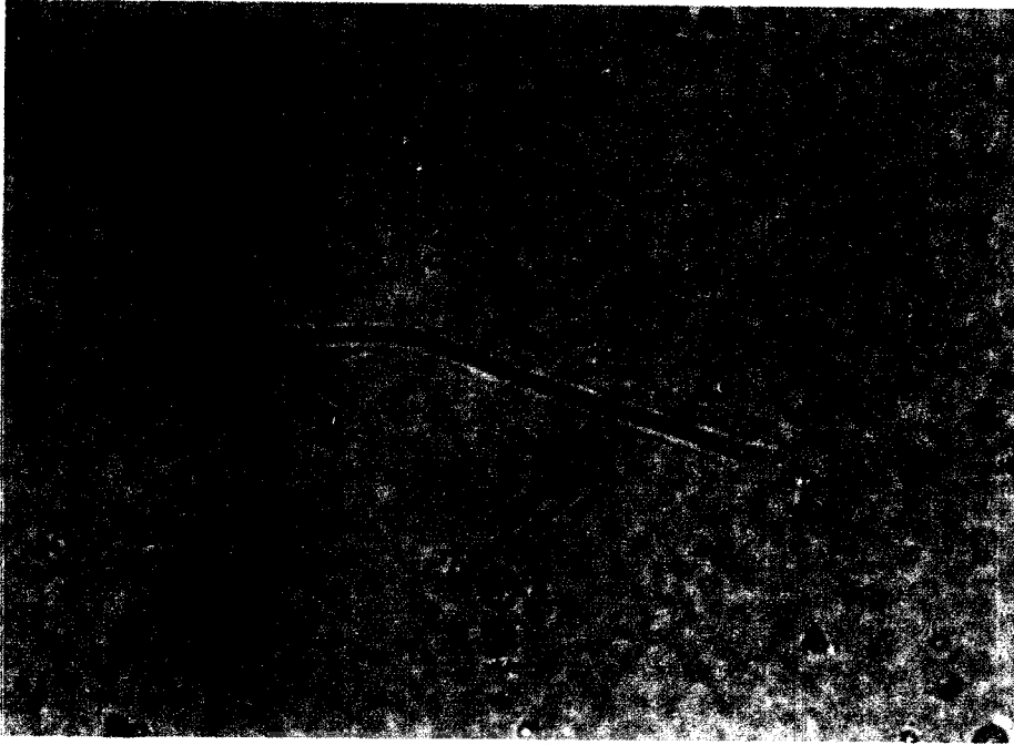
شکل شماره ۶: فتومیکروگراف از یک منفرد آزبست در نمونه هوای حوزه تنفسی در یک کارخانه آزبست - سیمان در بزرگنمایی 500 \times (طول لیف 37/0 \mu m ، قطر لیف: 1/0 \mu m و نسبت طول به قطر لیف: ۳۷).
